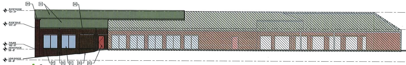
2 SOUTH EXTERIOR ELEVATION A3.1 SCALE: 1/8" = 1'-0"
