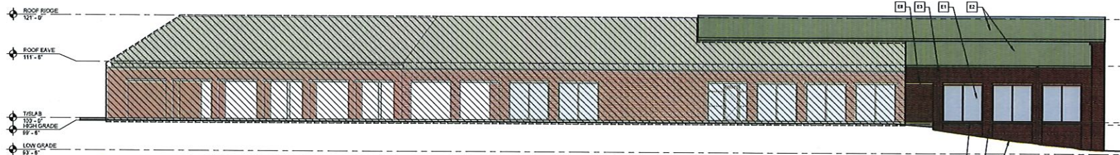
1 NORTH EXTERIOR ELEVATION A3.1 SCALE: 1/8" = 1'-0"
