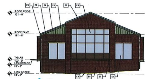
3 WEST EXTERIOR ELEVATION A3.1 SCALE: 1/8" = 1'-0"
