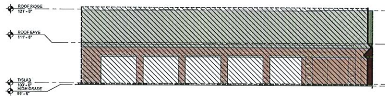
4 EAST EXTERIOR ELEVATION A3.1 SCALE: 1/8" = 1'-0"
